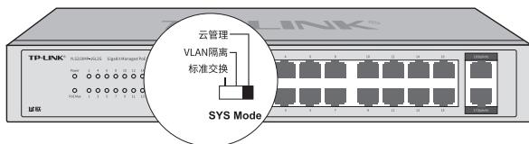
图1-10 系统模式选择开关示意图
