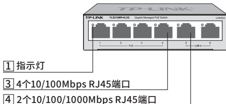
图1-2 前面板示意图
