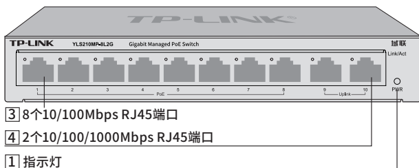
图1-4 前面板示意图
