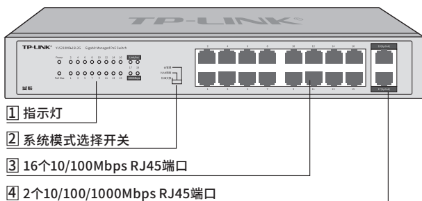
图1-6 前面板示意图
