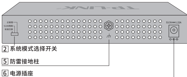
图1-5 后面板示意图
